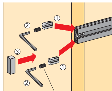
Madenschraube Eindrehmaß min. 6,5 mm
