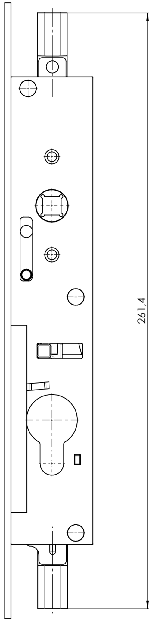
Darstellung verriegelt
