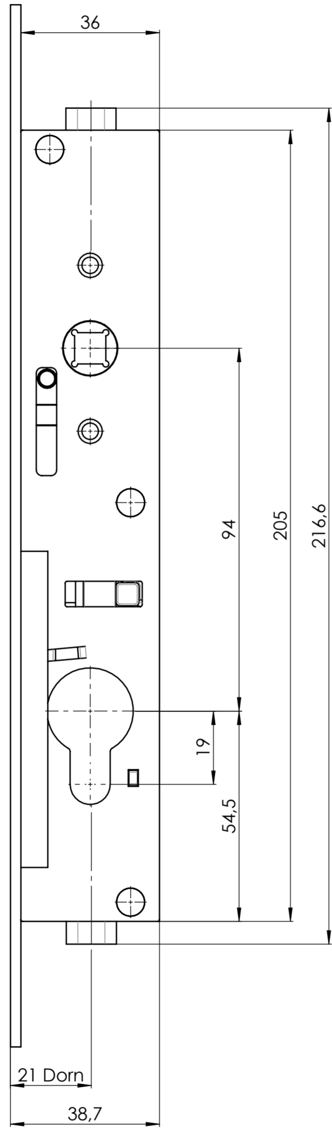
Darstellung geöffnet
